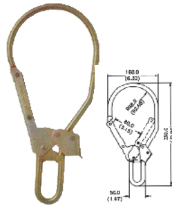
■ 11.344 Büyük Kanca 22 kN
