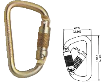
■ 11.340 Karabina Otomatik 22 kN
