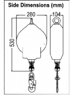
■ 11.504 Geri Sarım Makarası 25 mt
