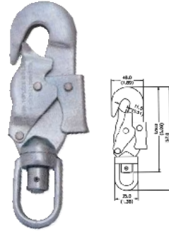
■ 11.342 Fırdöndü Kanca 22 kN
