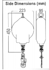
■ 11.502 Geri Sarım Makarası 15 mt
