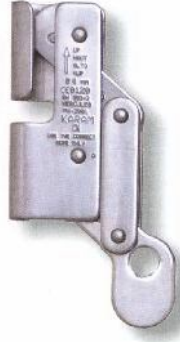
■ 11.552 Çelik Halat Tutucu
