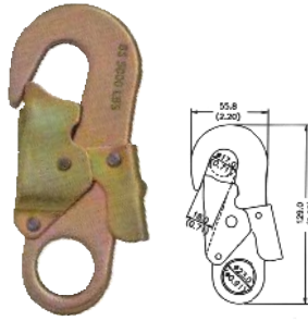
■ 11.341 Küçük Kanca Çift Emniyetli
