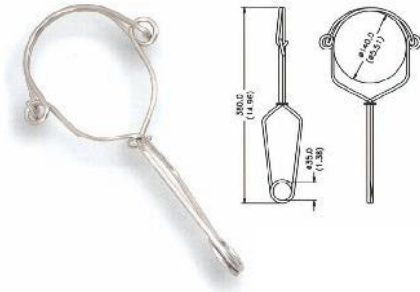
■ 11.545 Bağlantı Yayı 22 kN
